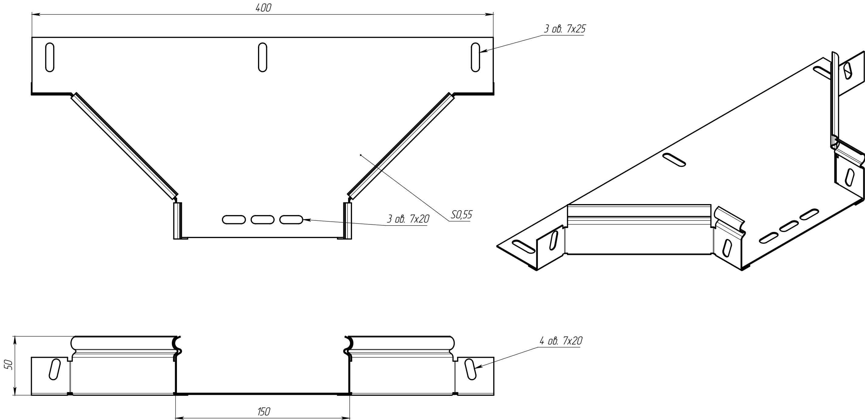
1. Размеры для справок
