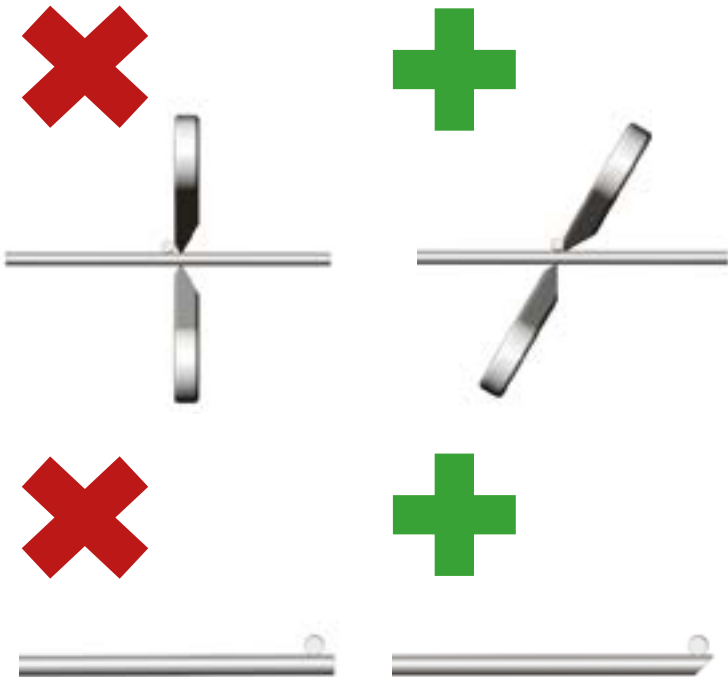
Примеры резки
